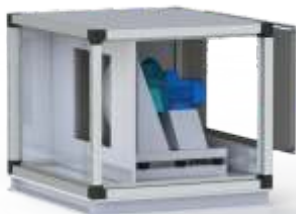
BPF 1/22-0,55(2) 2 полюсный электродвигатель [2; 4; 6; 8] Мощность двигателя 0,55кВт [0,37...45] Рабочее колесо 220мм [220...1100] 1 типоразмер [1...15] Вентиляторная секция
